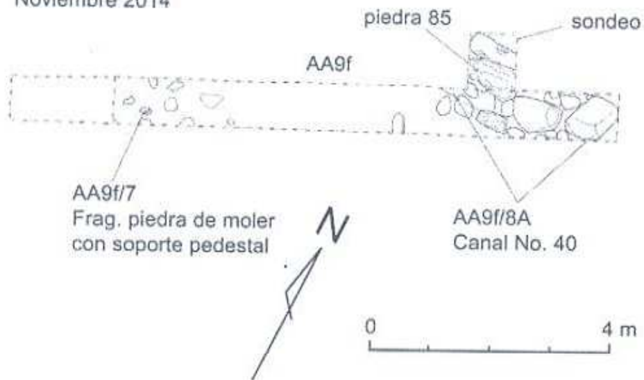
Figura 2. Planta del Canal No. 40 (AA9f/8A), Clásico Temprano Fase Alejos (150-300 DC), nótese la Piedra 85.
